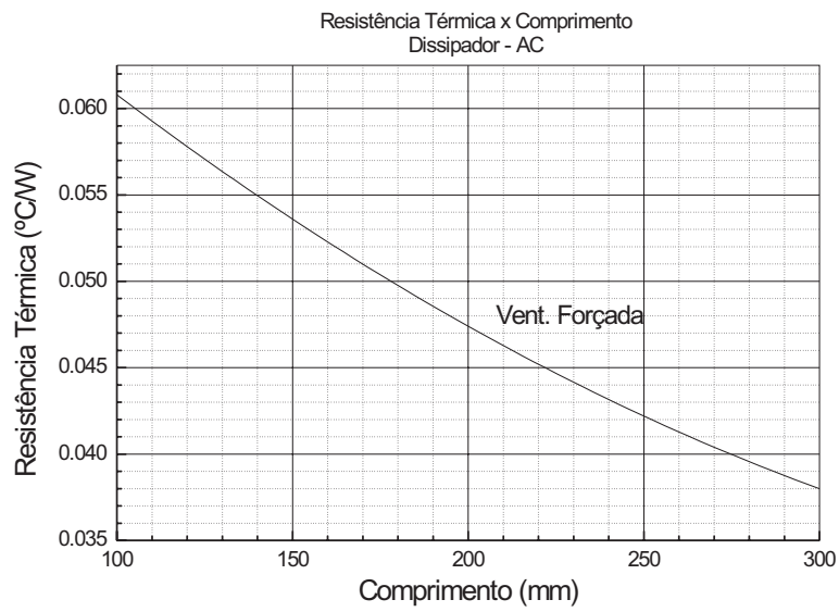
Fig.1 -Resistência térmica
