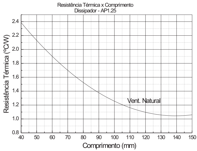
Fig.1 -Resistência térmica
